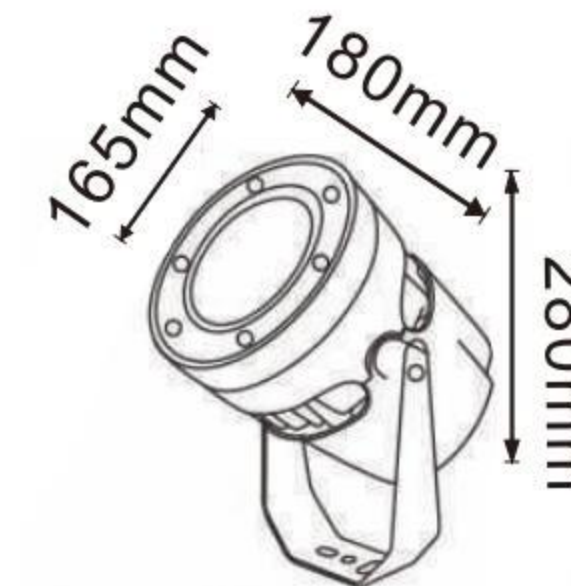
XYFLP-165-ZJ XYFLP-165H-ZJ
