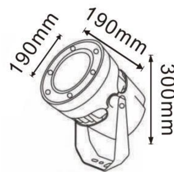
XYFLP-190-ZJ XYFLP-190H-ZJ
